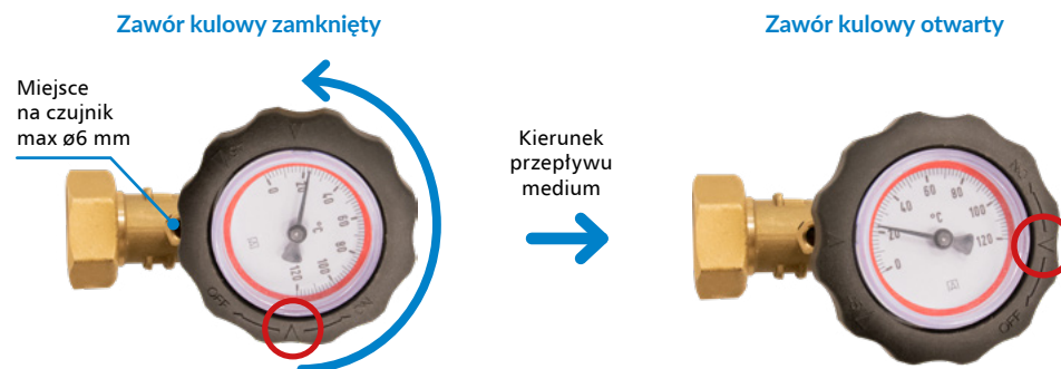
Rys. 2 Grupy pompowe BPS bez mieszania.
